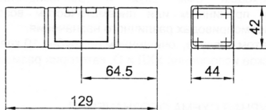
Размеры стыковой поверхности монтажной плиты
