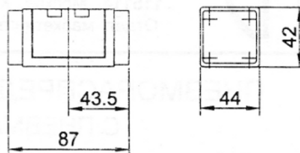
Пневмораспределители 5PM-6-311-0 и 5PM-6-312-0
