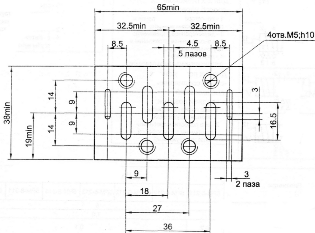
Размеры стыковой поверхности монтажной плиты
