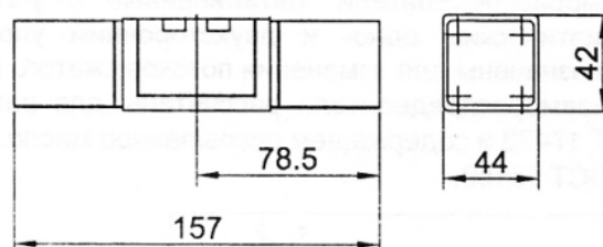
Пневмораспределители 5PM-6-311-0 и 5PM-6-312-0
