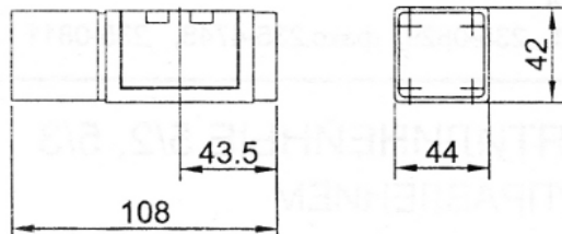
Пневмораспределитель 5PM-6-211-0, 5PM-6-213-0, 5PM-6-214-0
