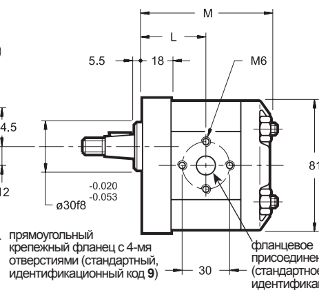
также имеются модели с резьбовыми отверстиями (идентификационный код B)
