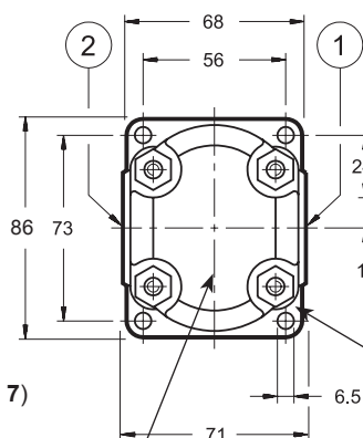
дренажный порт 1/4" BSP только на реверсивном насосе
