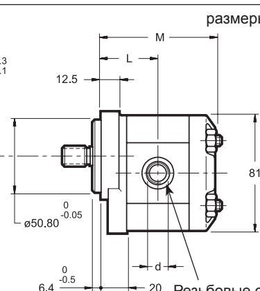
Резьбовые отверстия UNF (идентификационный код U)
