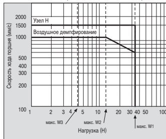
MY1M32 Горизонтальное столкновение; p=0.5 МПа
