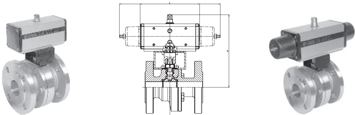
ATTUATORE PNEUMATICO DOPPIO EFFETTO (230 V ac) DOUBLE ACTING PNEUMATIC ACTUATOR
