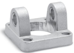
Передняя цапфа охватывающая Мод. H... и C-H...
