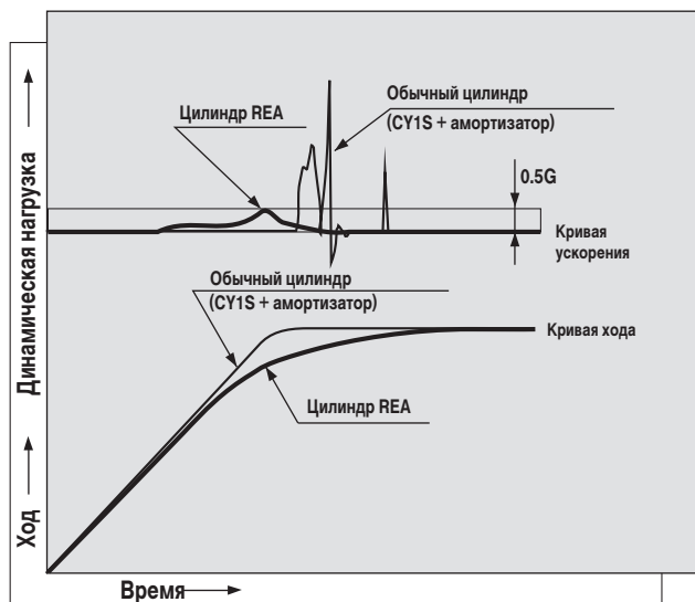
График, отражающий плавный разгон и торможение цилиндра:
