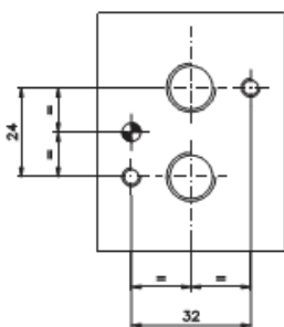
Размеры монтажной поверхности клапана NAMUR
